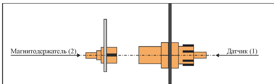
Рисунок 38 – Соосность датчика системы контроля
