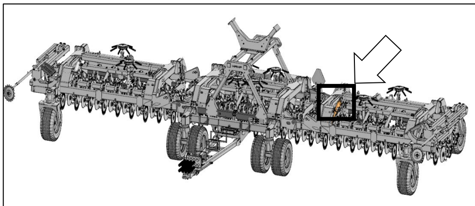
Рисунок 33 – Месторасположение гидравлического цилиндра
