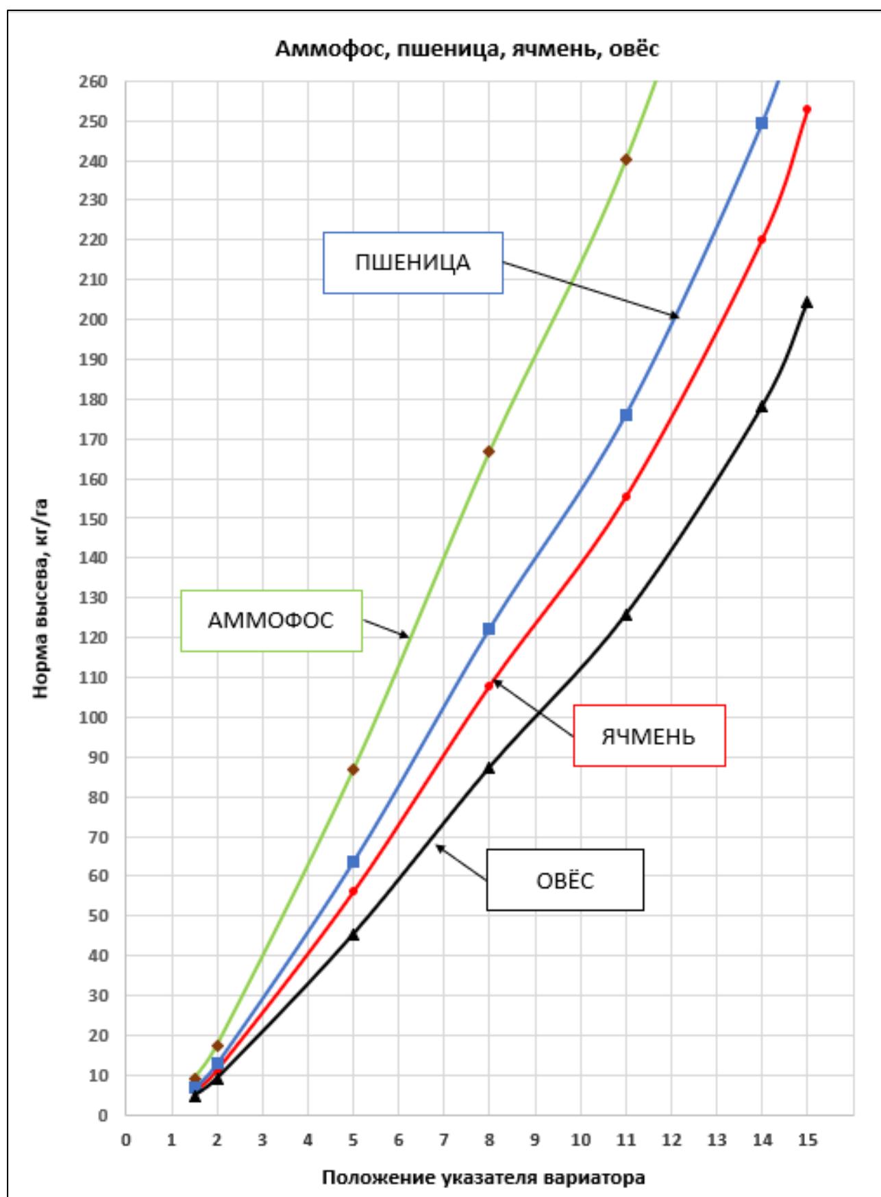
Рисунок 14 – Диаграмма ориентировочной нормы высева
