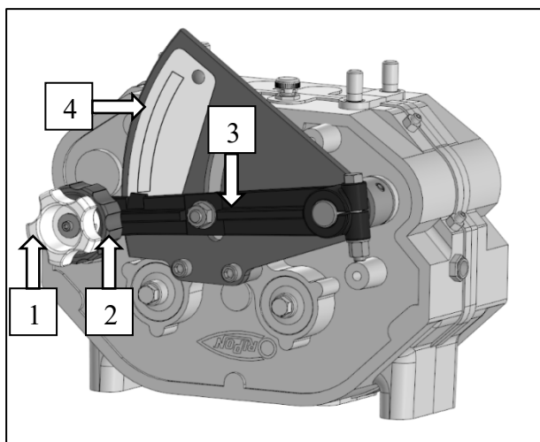
Рисунок 55 – Вариатор «ORIPON», «LASERKM»: 1 – Фиксатор регулятора; 2 – Регулятор; 3 – Указатель; 4 – Шкала вариатора
