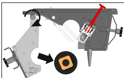
Рисунок 22 – Замена высевающего вала
