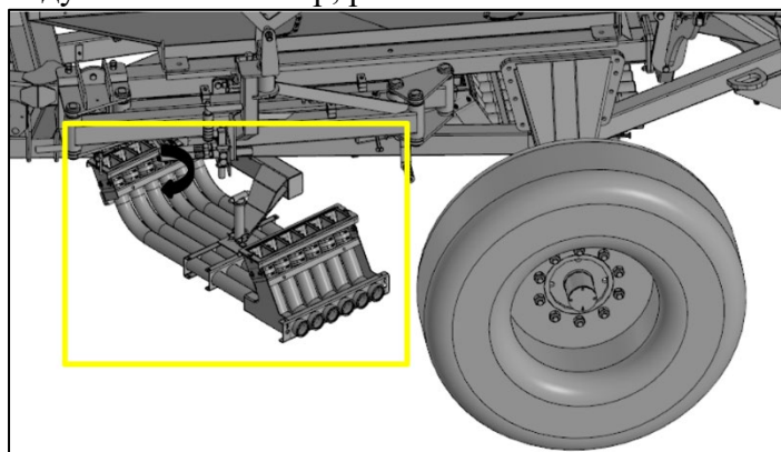
Рисунок 21 – Воздушный коллектор
