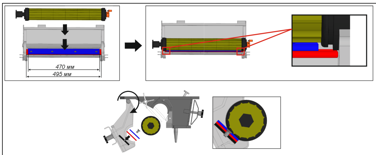
Рисунок 23 – Замена высевающего вала для мелкосемянных культур
