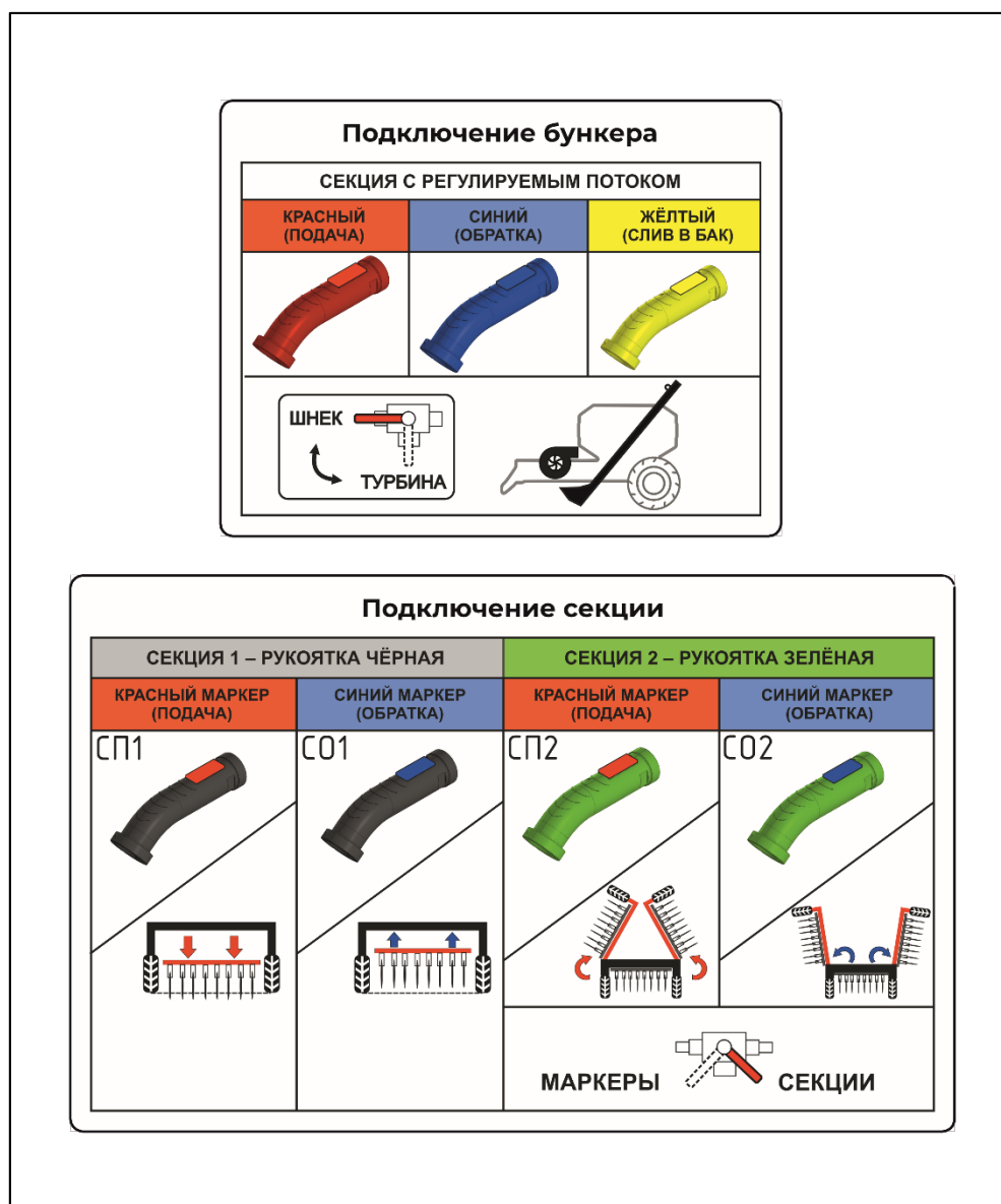
Рисунок 41 – Цветовая маркировка РВД (при наличии)
