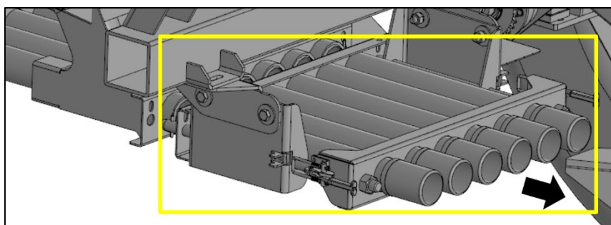
Рисунок 20 – Проставка воздушного коллектора
