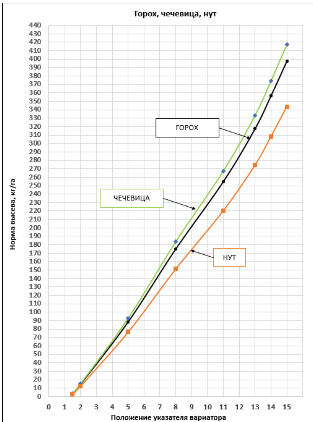
Рисунок 15 – Диаграмма ориентировочной нормы высева
