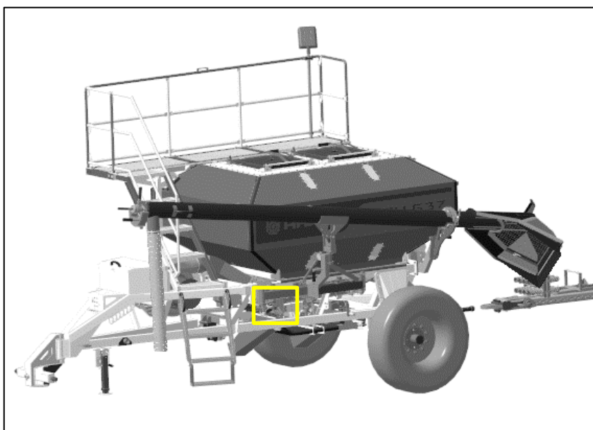
Рисунок 16 – Расположение рычага заслонки
