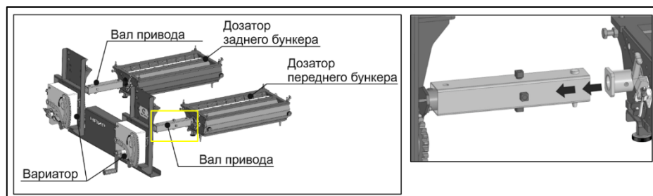
Рисунок 19 – Вал привода
