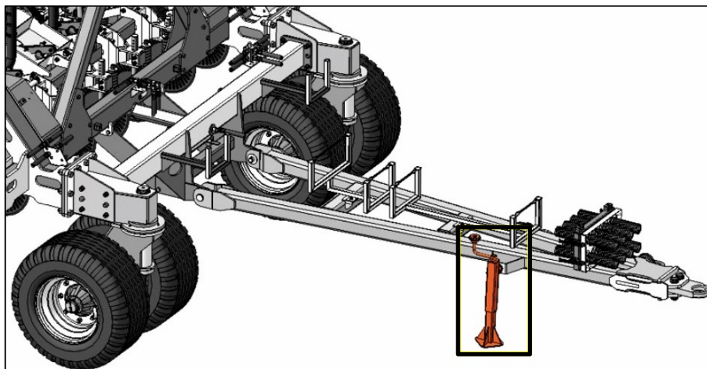
Рисунок 11 – Подножка рамы секции в рабочем положении
