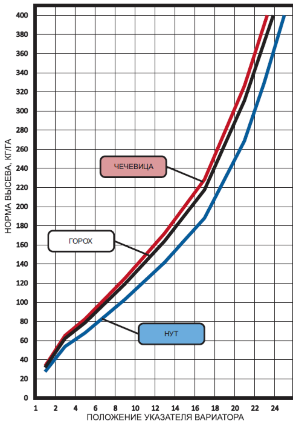
Рисунок 57 – Диаграмма ориентировочной нормы высева: Чечевица, горох, нут
