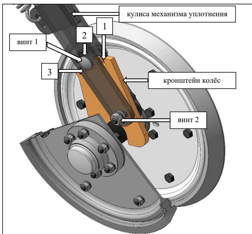
Рисунок 26 – Механизм уплотнения (вид в разрезе), 1,2,3 – пазы для фиксации кронштейна
