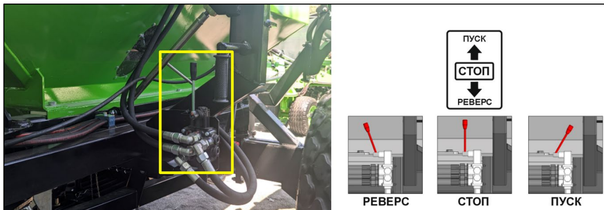
Рисунок 7 – Распределительный кран на шнеке
