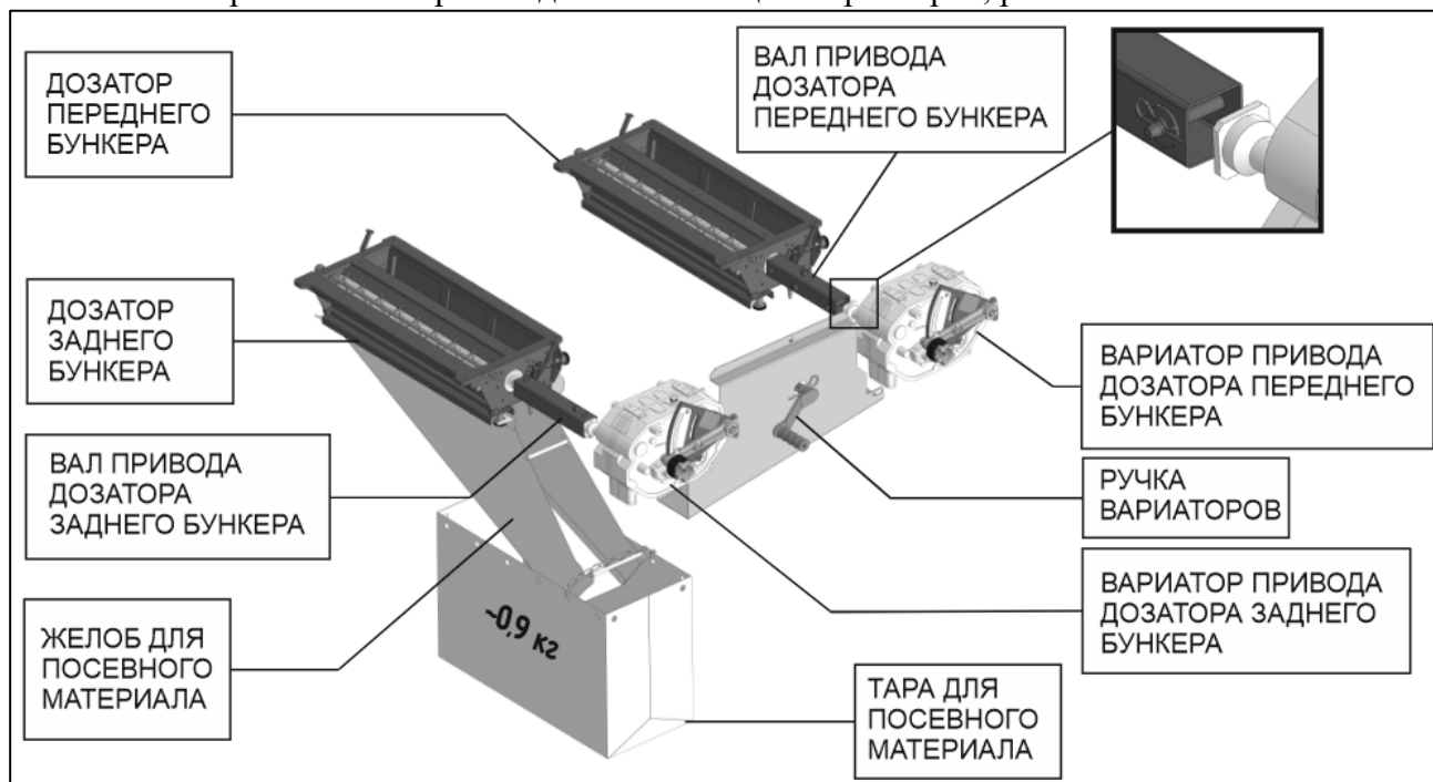
Рисунок 54 – Дозирующая система бункера с вариаторами «ORIPON», «LASERKM» (показана настройка дозатора заднего бункера)
