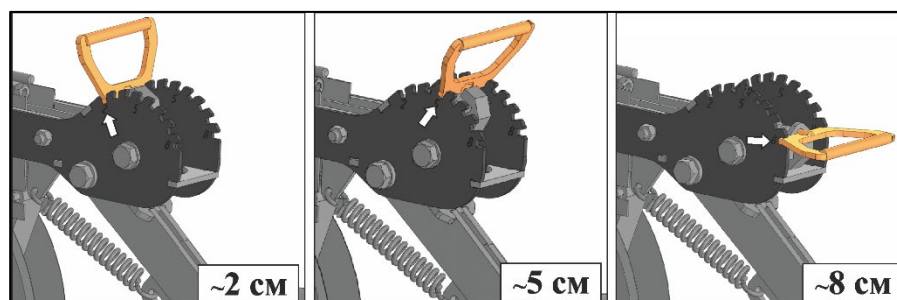
Рисунок 25 – Эксцентриковый упор
