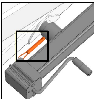
Рисунок 9 – Палец, фиксирующий подножку в транспортном положении
